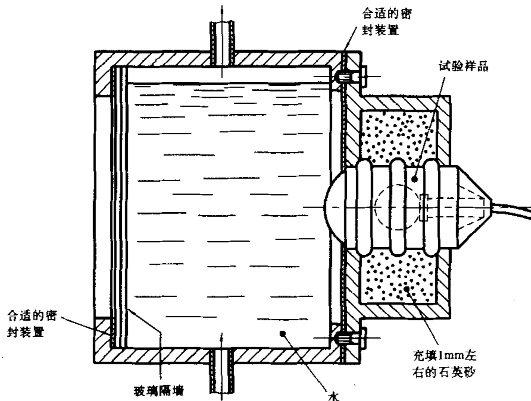
图 1 适合灯具前面跟水接触的试验装置
